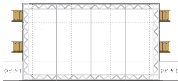
《上面図》
