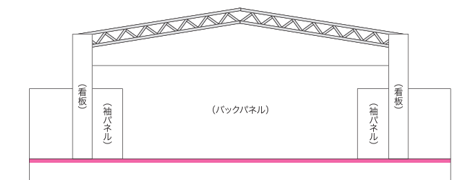
《正面図》
