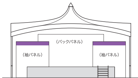
《正面図》
