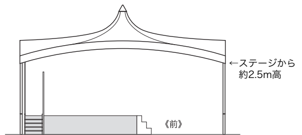
《側面図》
